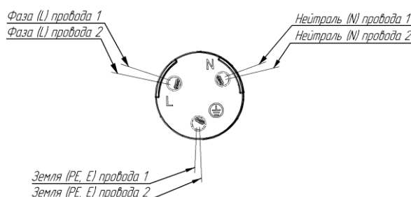
Контакты клеммы соединителя
